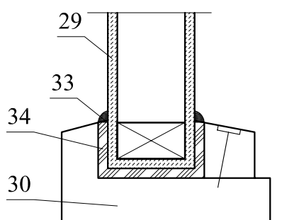
Узел "А-2"
