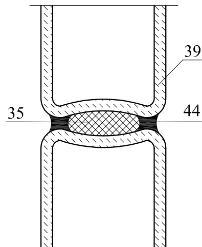
Узел "А"
