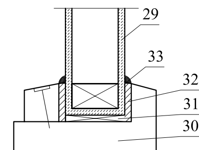
Узел "А-1"
