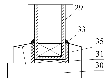
Узел "А-3"
