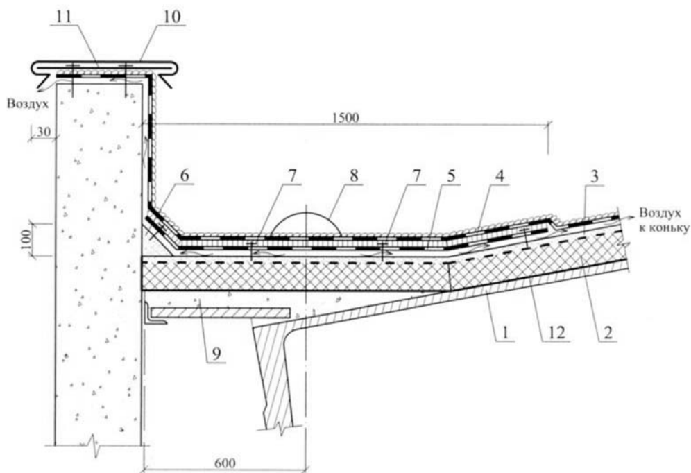
Рис. 11. Примыкание водоизоляционного слой к парапету
