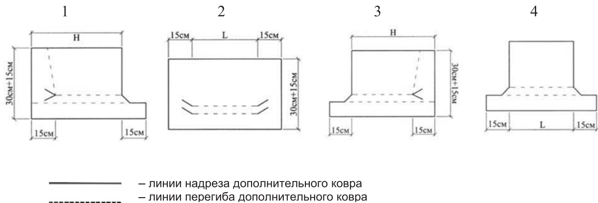
Рис. 14. Раскрой рулонного материала по сторонам трубы 1, 3 – боковые стенки трубы; 2 – передняя стенка трубы; 4 – задняя стенка трубы
